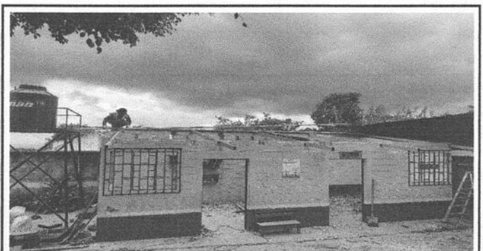
Foto 6: instalación de estructura de techo a modulo de trabajo numero 3, dirección y bodega.
