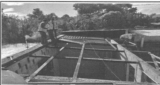
Foto 5: Destechado y sustitución de estructura de madera de techo de modulo de trabajo numero 3, dirección y bodega
