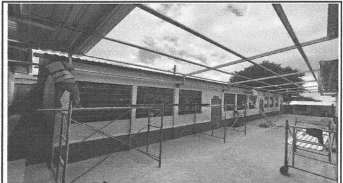
Foto 4: instalación de canales y bajada pluviales, inicio de instalación de techo, modulo de trabajo numero 2.
