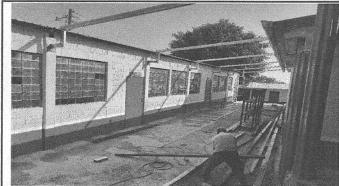
Foto 3: elaboración de estructura de techo del corredor, modulo de trabajo numero 2.
